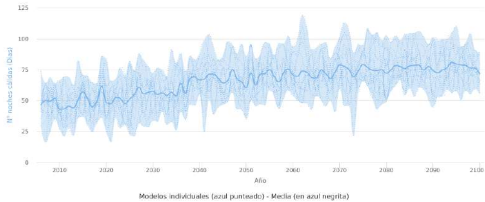
Gráfico 20: N° de noches cálidas en Cabra (2006-2100). RCP 4.5.
