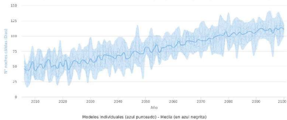
Gráfico 21: N° de noches cálidas en Cabra (2006-2100). RCP 8.5.
